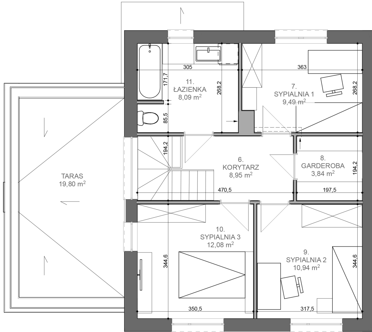
RZUT PIĘTRA
