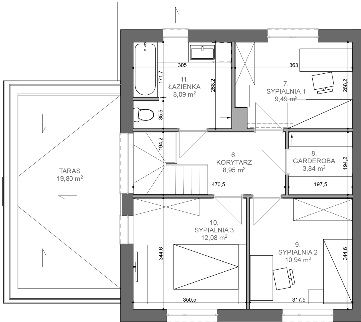
RZUT PIĘTRA
